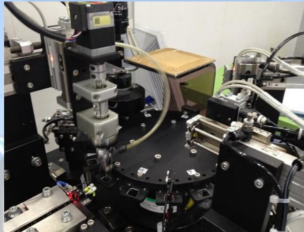
画像検査機
